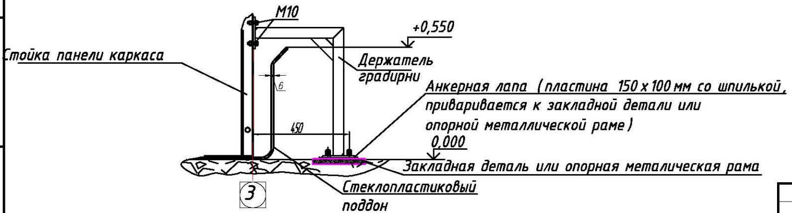
Р-Р Установка держателя грядирни
