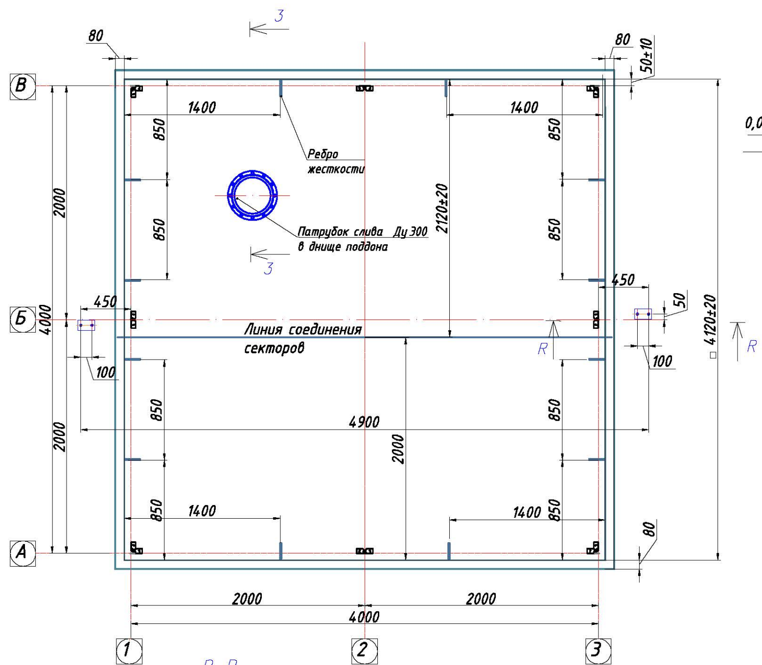
Р-Р Установка держателя грядирни
